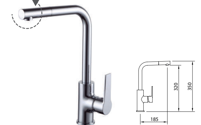
Mezclador con aireador, caño giratorio, flexibles M-10 3/8" x 370 mm. Mixer with aerator, swivel spout, flexible hoses M-10 3/8" x 370 mm. Mitigeur évier bec orientable, aérateur, raccords flexibles M-10 3/8" x 370 mm
