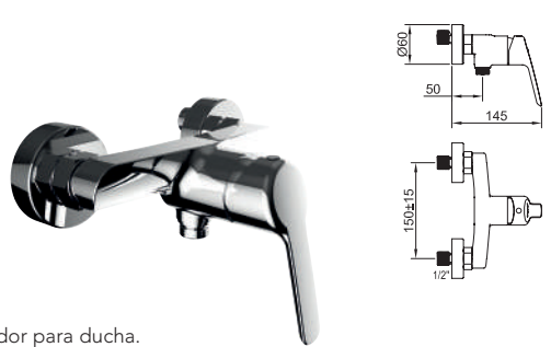
Mezclador para ducha. Shower mixer. Mitigeur douche
