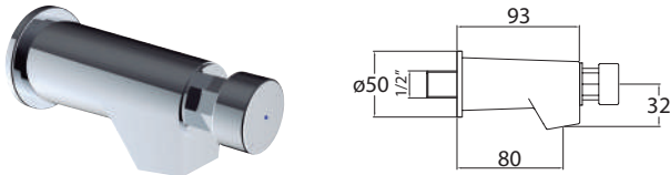
Grifo mural para lavabo, con aireador, <14 segundos, cartucho M28 Wall mounted basin tap, with aerator, <14 seconds, cartridge M28 Robinet simple, avec aérateur, <14 secondes cartouche M28
