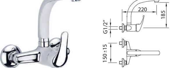
Mezclador con aireador, caño conformado giratorio. Mixer with aerator, swivel tube spout. Mitigeur évier mural, bec orientable façonné, aérateur
