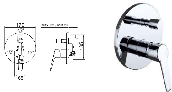
Mezclador empotrable de 1/2" para baño-ducha, inversor automático Concealed bath-shower mixer 1/2", automatic diverter Mitigeur encastré, 1/2", inverseur automatique
