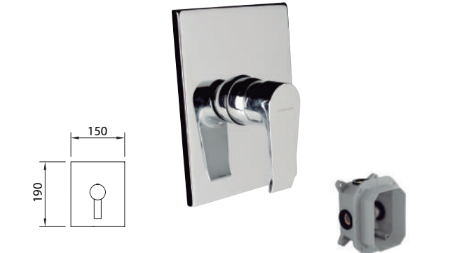
Mezclador empotrable de 1/2" para ducha Concealed shower mixer 1/2" Mitigeur encastré, 1/2"
