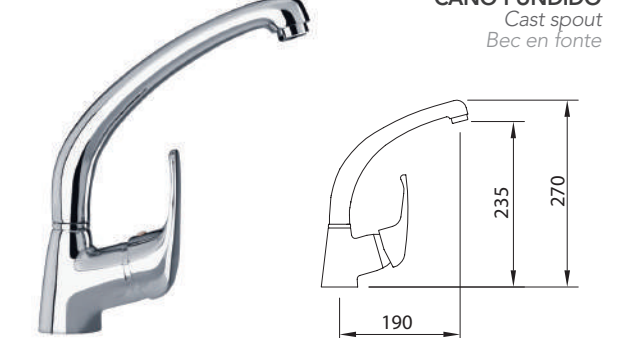
Mezclador con aireador, caño fundido giratorio, flexibles M-10 3/8" x 370 mm. Mixer with aerator, swivel cast spout, flexible hoses M-10 3/8" x 370 mm. Mitigeur évier bec orientable, aérateur, raccords flexibles M-10 3/8" x 370 mm
