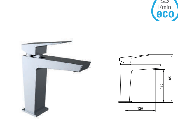
LAVABO 130 Basin mixer 130 / Mitigeur lavabo 130
