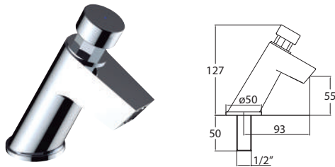
Grifo de repisa para lavabo, con aireador, <14 segundos, cartucho M28 Deck mounted basin tap, with aerator, <14 seconds, cartridge M28 Robinet simple, avec aérateur, <14 secondes cartouche M28
