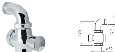
Fluxor exterior para sanitario. Restroom external fluxor. Robinet temporisé sanitaire mural.
