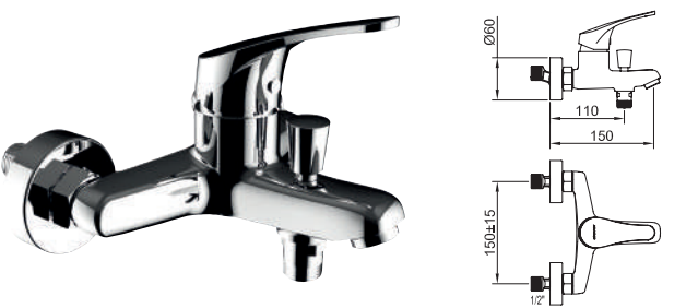
Mezclador con aireador baño-ducha, inversor automático. Bath-shower mixer with aerator, automatic diverter. Mitigeur bain-douche, aérateur, inverseur automatique
