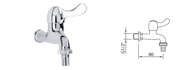
Grifo de pared. Accesorio manguera. Wall mounted single tap. Hose fitting. Robinet, aérateur. Raccord pour tuyau.
