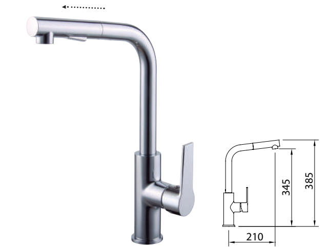
Mezclador con aireador, caño giratorio, ducha extraíble con pulsador para lavavajillas, enlaces de alimentación flexibles M-10 3/8" x 370 mm. Mixer with aerator, swivel spout, pull-out handset and flexible hoses M-10 3/8" x 370 mm. Mitigeur évier bec orientable, aérateur, douchette extractible avec poussoir pré-lavage, raccords flexibles M-10 3/8" x 370 mm
