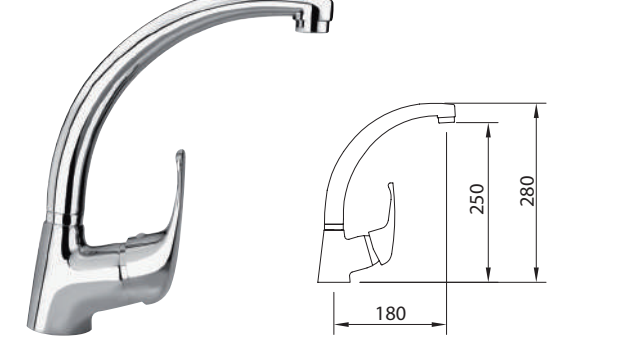
Mezclador con aireador, caño conformado giratorio, flexibles M-10 3/8" x 370 mm. Mixer with aerator, swivel tube spout, flexible hoses M-10 3/8" x 370 mm. Mitigeur évier bec orientable, aérateur, raccords flexibles M-10 3/8" x 370 mm
