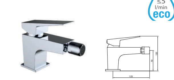
BIDÉ 70 Bidet mixer / Mitigeur bidet
