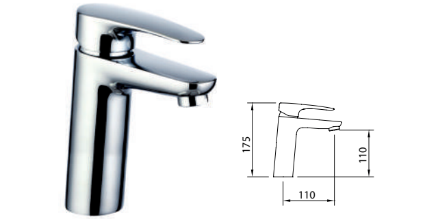
LAVABO 110 / Basin mixer 110 / Mitigeur lavabo 110
