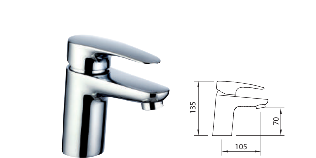
LAVABO 70 / Basin mixer 70 / Mitigeur lavabo 70
