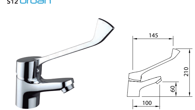
LAVABO CON MANETA GERONTOLÓGICA / Basin mixer with medical lever / Mitigeur lavabo avec manette médicale
