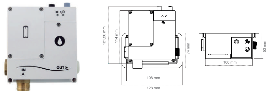
Caja estándar con platina sujeción pared incluida. Para 60739-60740. Standard box with enclosure wall included. For 60739-60740. Boîtier standard avec platine de fixation murale incluse. Pour 60739-60740.
