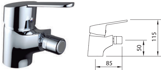
Mezclador con aireador a rótula y flexibles M-10 3/8" x 370 mm. Mixer, swivel aerator, flexible hoses M-10 3/8" x 370 mm. Mitigeur bidet, aérateur rotule, raccords flexibles M-10 3/8" x 370 mm
