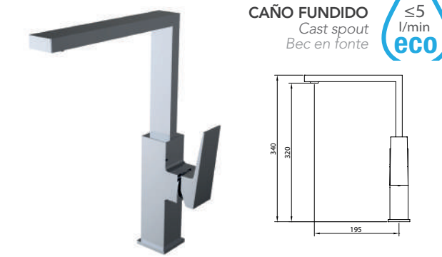
FREGADERO Sink mixer / Mitigeur évier
