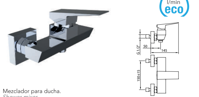
DUCHA Shower mixer / Mitigeur douche
