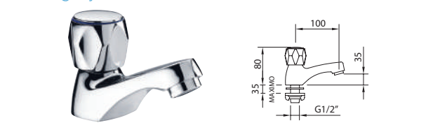
Grifo de repisa, con aireador, índice de agua fría. Deck mounted single basin faucet, with aerator, cold water indice. Robinet, aérateur
