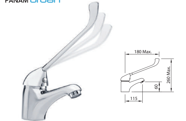
LAVABO CON MANETA GERONTOLÓGICA / Basin mixer with medical lever / Mitigeur lavabo avec manette médicale
