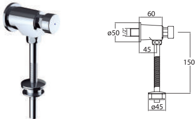
Grifo mural de 1/2" para urinario, 7 segundos, cartucho M28. Urinal 1/2", 7 seconds, cartridge M28. Robinet temporisé urinoir 1/2", 7 secondes, cartouche M28.
