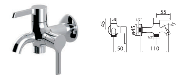
Grifo de pared salida fregadero / lavadero / lavadora. Wall mounted single tap. Robinet, aérateur
