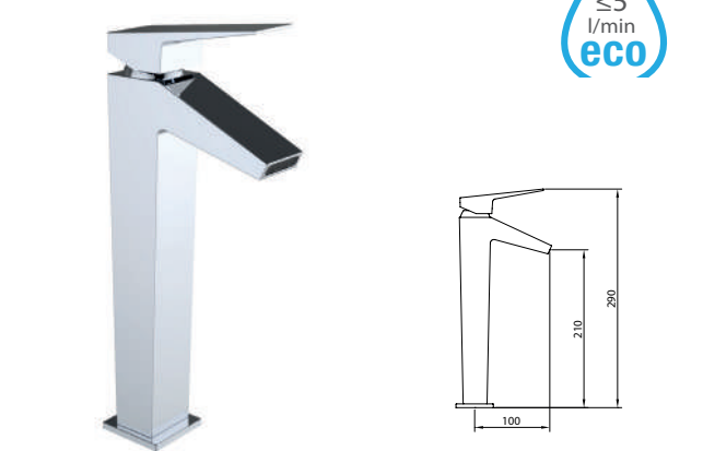
LAVABO 210 Basin mixer 210 / Mitigeur lavabo 210
