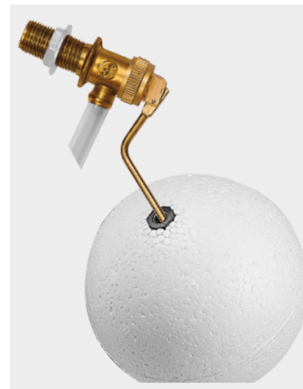
GPB 2 Ref. 0151551530 Packaging Bolsa 25 uds/caja PVP: 11,52 € Grifo lateral (Latón) + Tuerca (Plástico) + Boya Ø 3/8" Latón + Longitud: 32 mm
