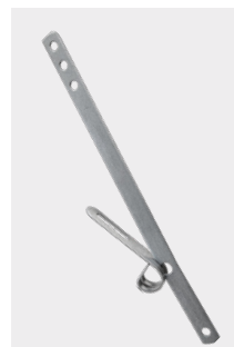
Palanca PA 30 Ref. 0154007030 Granel 25 uds/caja PVP: 1,14 € Longitud: 300 mm
