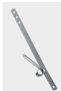
Palanca PA 27 Ref. 0154007020 Granel 25 uds/caja PVP: 1,23 € Longitud: 275 mm
