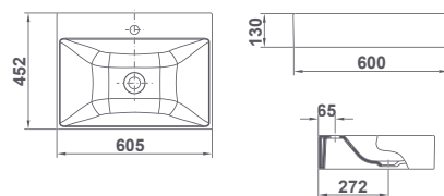
10215 ALBUS 60 x 45 cm Sin rebosadero. Con orificio de grifería. Esmaltado por los cuatro lados.
