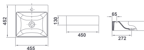
10219 ALBUS 45 x 45 cm Sin rebosadero. Con orificio de grifería. Esmaltado por los cuatro lados.
