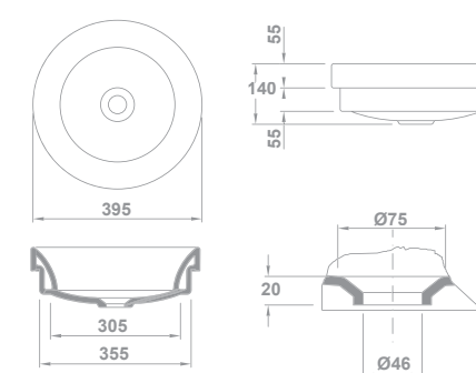
04330 CIRCLE Ø 39,5 cm Sin rebosadero. Sin orificio de grifería. Posibilidad de instalación sobre-encimera, encimera o semiempotrar. Plantilla de corte de Ø 31,2 cm para instalación sobre-encimera.
