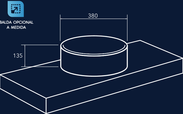
TECNICO SOBRE ENCIMERA Medidas expresadas en milímetros
