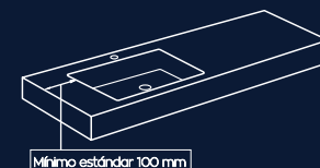
Mínimo estándar 100 mm FALDÓN SENO DESPLAZADO desde 800 mm
