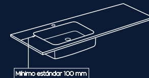
Mínimo estándar 100 mm MUEBLE SENO DESPLAZADO desde 800 mm (enviar cotas del mueble)
