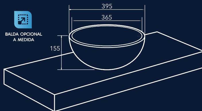
TECNICO SOBRE ENCIMERA Medidas expresadas en milímetros
